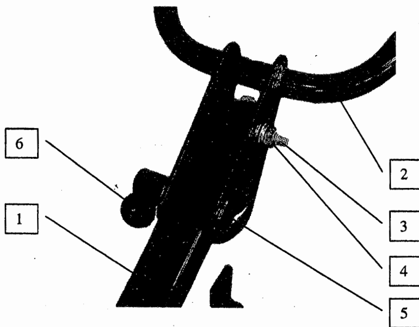
Рисунок 3 – Схема присоединения руля к рулевой колонки
